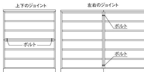
本体内部図 (引出しを抜いた図)
